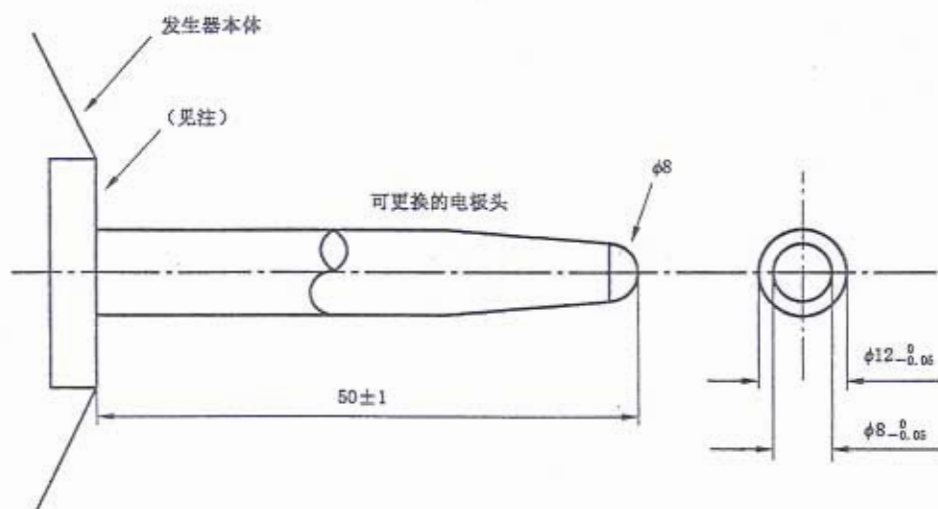
a) 空气放电
